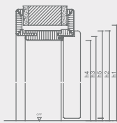
Vertikalschnitt Futter (RF)
