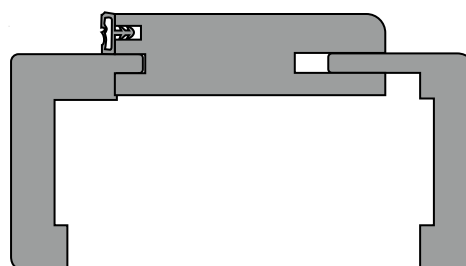
ZARGE MIT KLEINER RUNDKANTE CADRE AVEC PETIT CHANT ARRONDI
