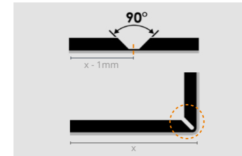
Fräsnut 90° - Beispiel
