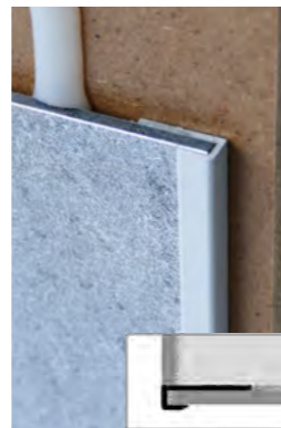
Abschlussprofil Typ 800 U
