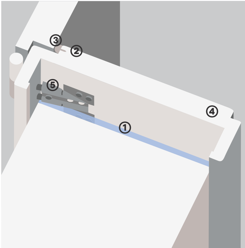
Optimierte Zargenkonstruktion mit neuer abgeschrägter Aufschraubbandtasche
