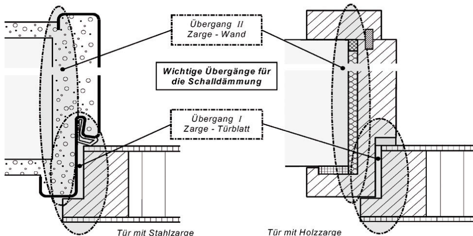
Bild 7 Wichtige Abdichtungsbereiche bei Türen
