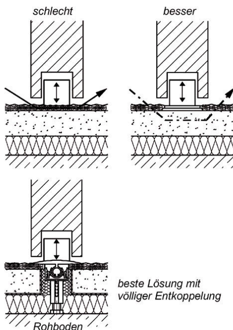
Bild 10 Schallübertragungswege u. Entkoppelungsmaßnahmen im Fußbodenanschlussbereich
