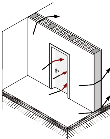
Bild 3 Schallübertragungswege bei einer Trennwand mit Verbindungstür
