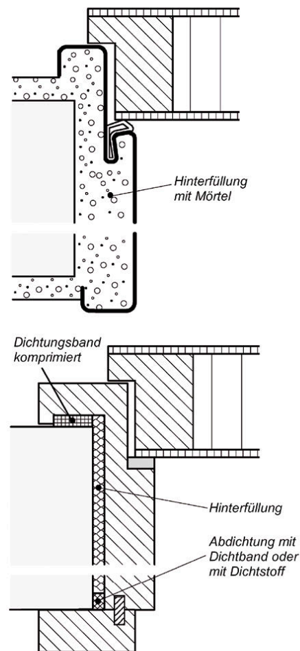
Bild 11 Hinterfüllungs- und Abdichtungsmaßnahmen an Türzarge
