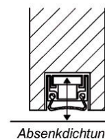
Bild 9 Abdichtungsmöglichkeiten zwischen Tür und Fußboden
