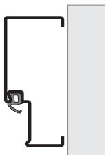
Blockzarge Typ 1 Einbau in der Öffnung E-Typ 1
