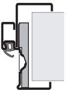
Eckzarge Diagonalbefestigung mit Ergänzungszarge Vario B53 C-Typ 1
