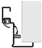
Eckzarge Diagonalbefestigung (mit Gewindebolzen) A-Typ 2
