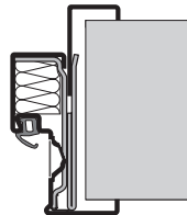
DryFix-Zarge mit Ergänzungszarge Vario B36 B-Typ 2
