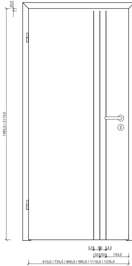
Ansicht "V-Fuge"
