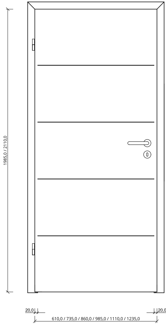
Ansicht "V-Fuge"
