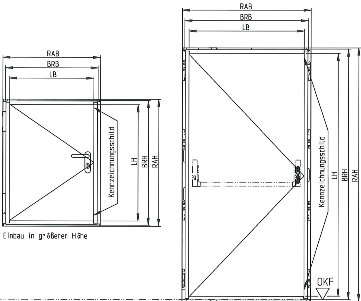
Ansicht Schließseite
